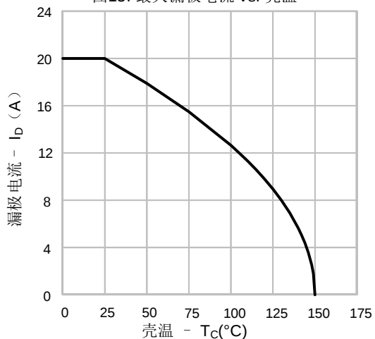
图13. 最大漏极电流 vs. 壳温
