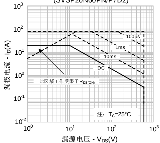
图12-3. 最大安全工作区域 (SVSP20N60PN/P7D2)
