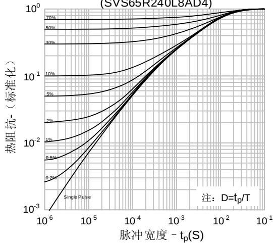
图16-3. 瞬态热阻抗 vs. 脉冲宽度 (SVS65R240L8AD4)
