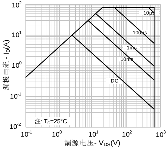
图 13-3. 最大安全工作区域(SVS65R240L8AD4)
