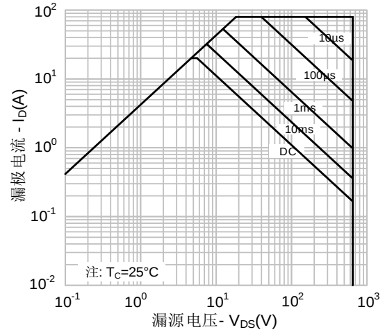
图 13-4. 最大安全工作区域(SVS65R240TD4)
