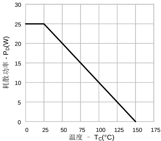
图14-1. 耗散功率 vs. 温度(SVS65R240FJD/FD4)
