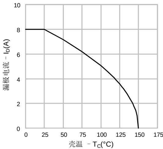
图15.漏极电流 vs. 壳温
