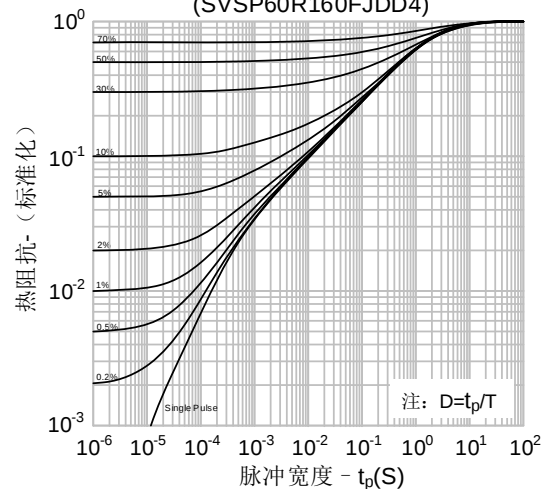
图16-1.瞬态热阻抗 vs. 脉冲宽度 (SVSP60R160FJDD4)
