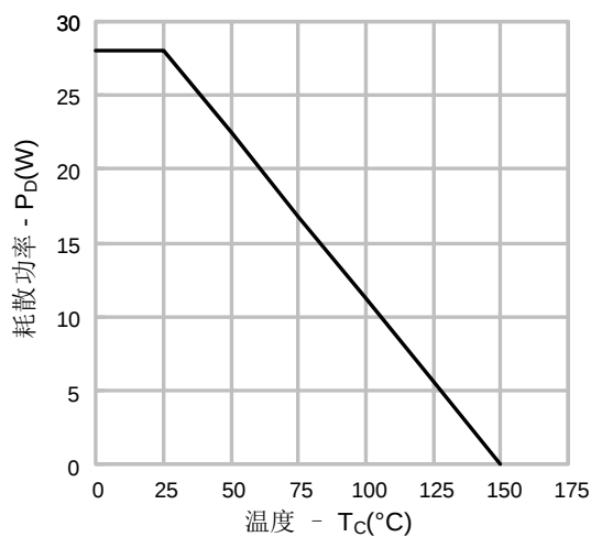
图14-1. 耗散功率vs.温度(SVSP60R160FJDD4)
