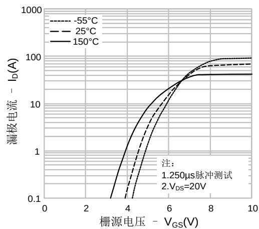
图 3. 传输特性
