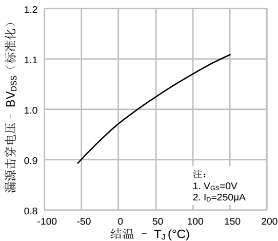
图 11. 击穿电压vs.温度特性
