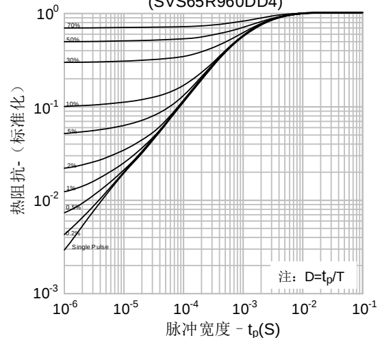
图16-1.瞬态热阻抗 vs. 脉冲宽度 (SVS65R960DD4)
