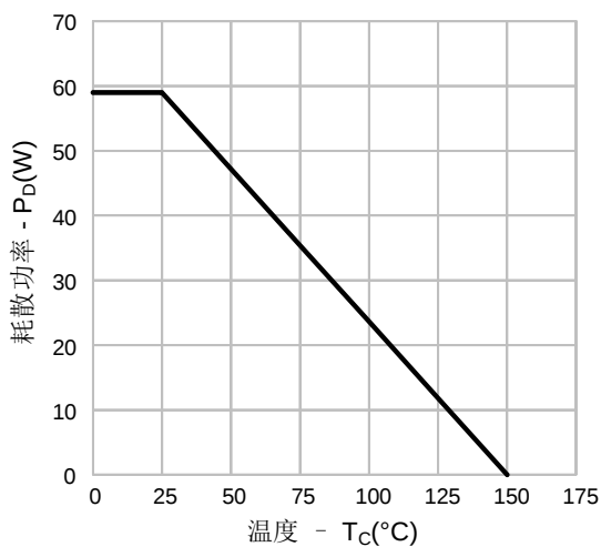
图14-1. 耗散功率vs.温度(SVS65R960DD4)
