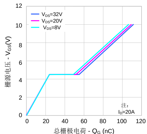
图 6. 电荷量特性
