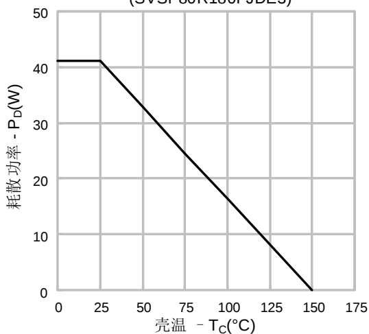
图14-2. 耗散功率vs.温度 (SVSP80R180FJDE3)
