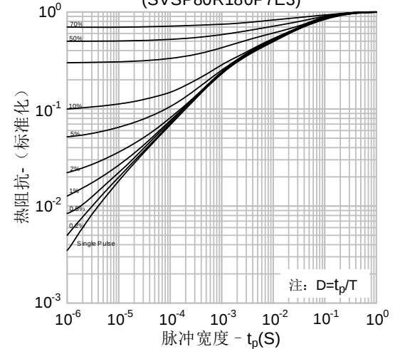
图16-3.瞬态热阻抗 vs. 脉冲宽度 (SVSP80R180P7E3)
