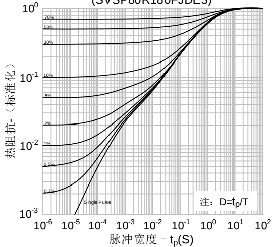
图16-2.瞬态热阻抗 vs. 脉冲宽度 (SVSP80R180FJDE3)
