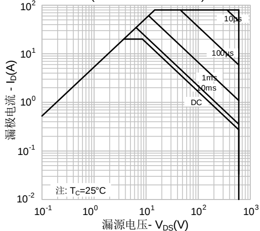
图 13-5. 最大安全工作区域 (SVSP60R190L8AD4)
