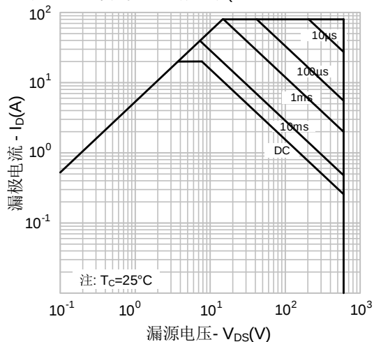
图 13-5. 最大安全工作区域 (SVSP60R190L8AD4)
