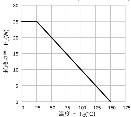
图14-1. 耗散功率vs.温度(SVSP60R190FJDD4)
