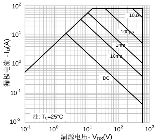
图 13-3. 最大安全工作区域(SVSP60R190T/KD4)
