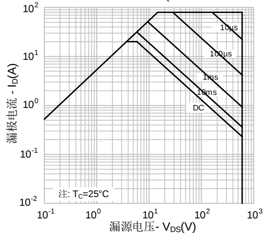
图 13-4. 最大安全工作区域(SVSP60R190P7D4)
