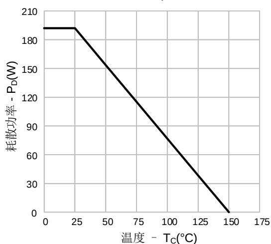
图14-3. 耗散功率vs.温度(SVSP65R135L8AD4)
