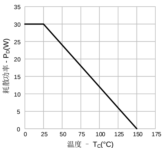
图14-2. 耗散功率vs.温度(SVSP65R135FJDD4)
