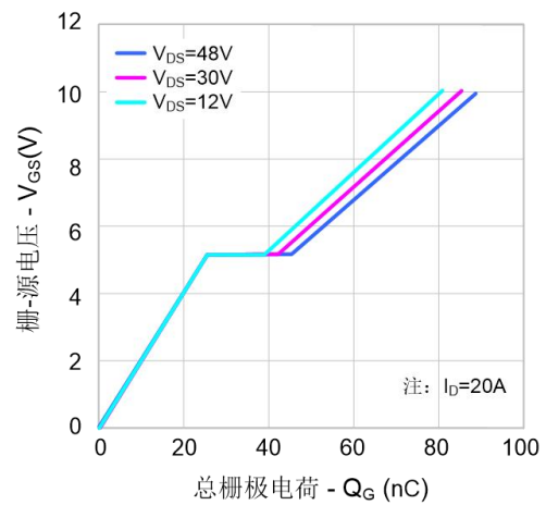
图 6. 电荷量特性
