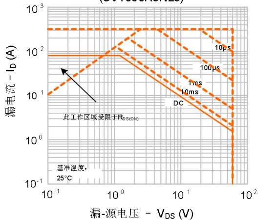
图 9-3. 最大安全工作区域 (SVT068R5NL5)
