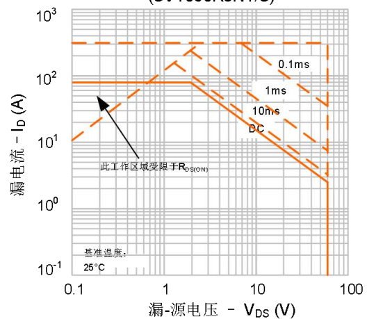
图 9-2. 最大安全工作区域 (SVT068R5NT/S)
