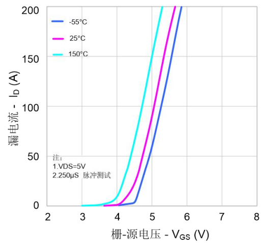
图 2. 传输特性
