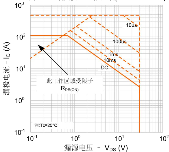
图 11-1. 最大安全工作区域(SVT034R6ND)
