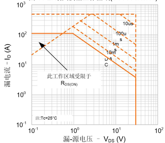
图 11-2. 最大安全工作区域(SVT034R6NT)
