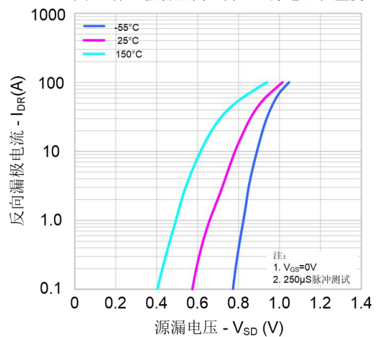
图 6. 体二极管正向压降 vs. 源电流和温度
