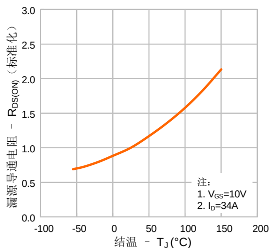
图 12. 导通电阻 vs. 温度特性
