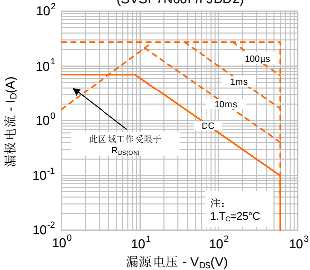
图9-1. 最大安全工作区域 (SVSP7N60F/FJDD2)
