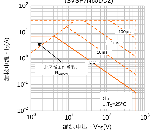
图9-2. 最大安全工作区域 (SVSP7N60DD2)
