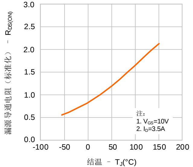
图8. 导通电阻 vs. 温度特性
