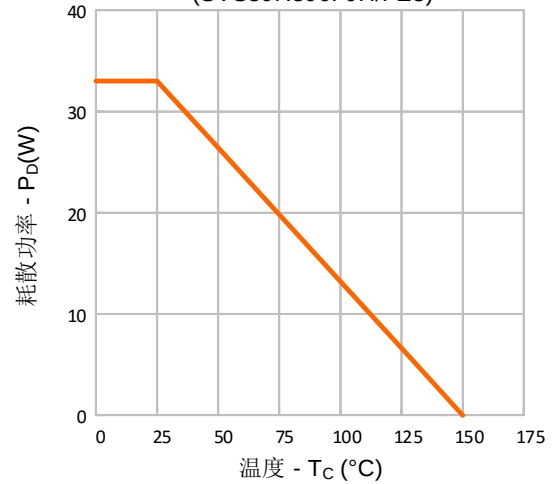
图 13-1. 耗散功率VS.温度 (SVS80R800FJH/FE3)
