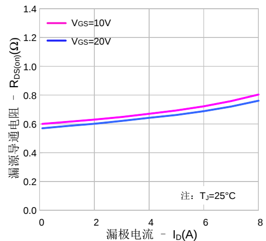
图 4. 导通电阻 vs. 漏极电流
