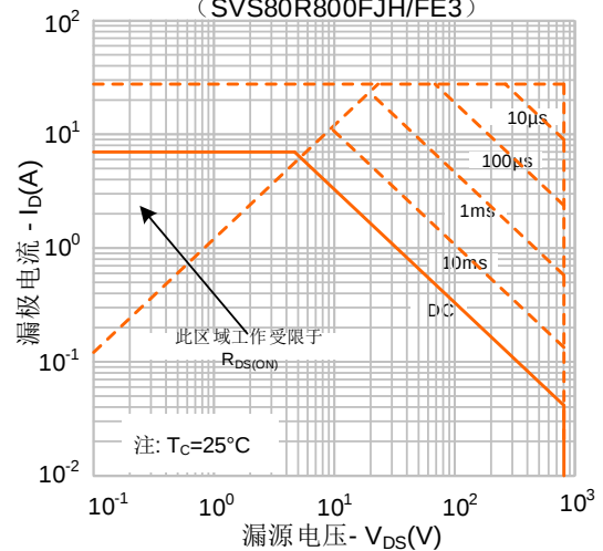
图 12-1. 最大安全工作区域 (SVS80R800FJH/FE3)
