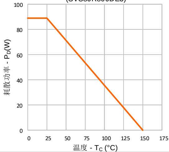
图 13-2. 耗散功率VS.温度 (SVS80R800DE3)
