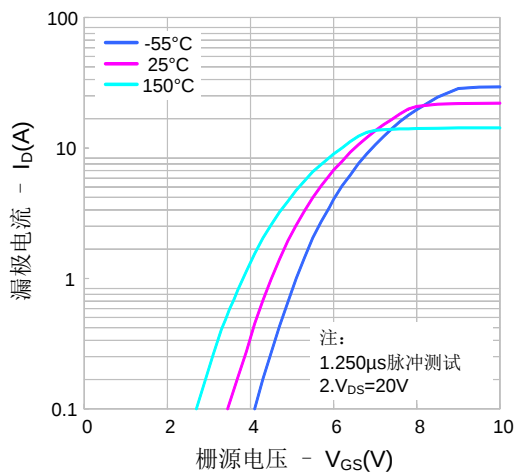
图 3. 传输特性
