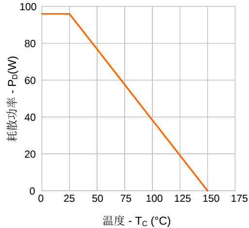
图13-3. 耗散功率vs.温度 (SVS70R420F/FJH/FJDE3)
