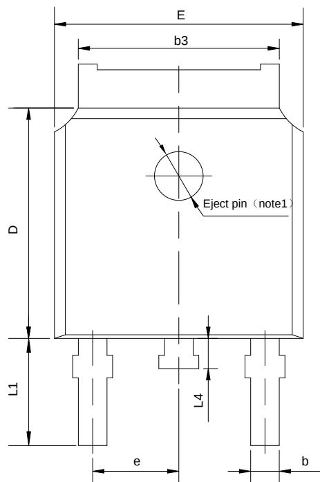
TO-263-2L
