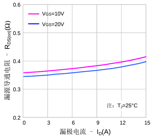
图 4. 导通电阻vs.漏极电流
