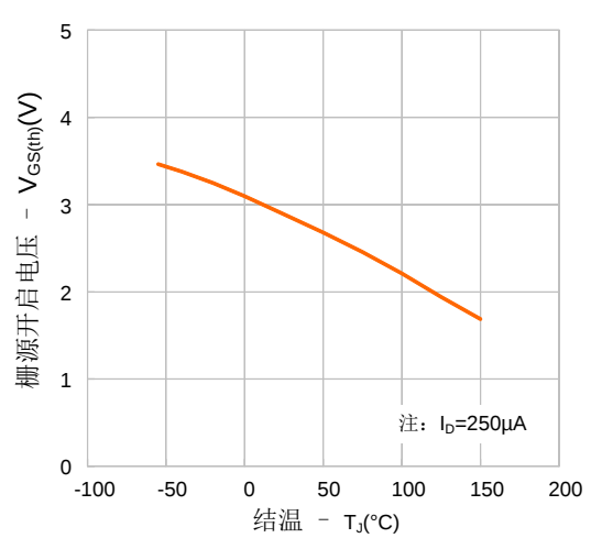
图 6. 开启电压vs.温度特性
