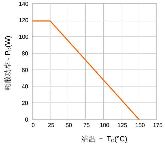
图13-2. 耗散功率vs.温度(SVS70R420SE3)
