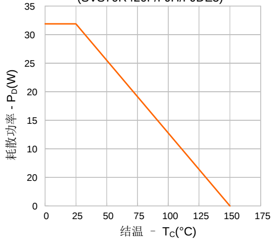
图13-3. 耗散功率vs.温度 (SVS70R420F/FJH/FJDE3)
