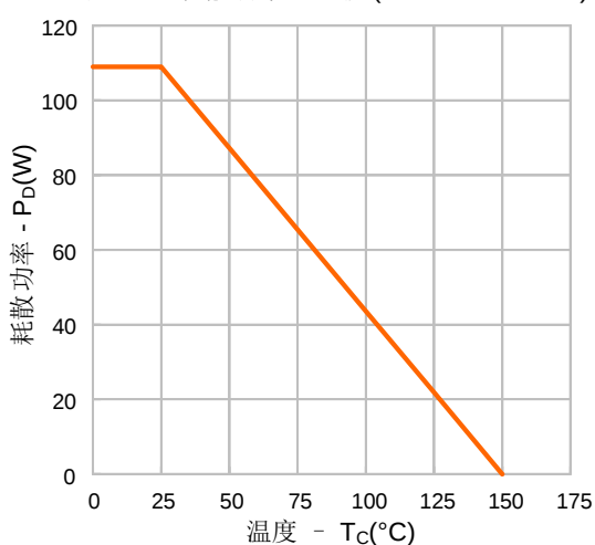
图14-2. 耗散功率vs.温度(SVS65R280DD4)
