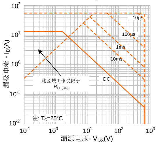
图 13-3. 最大安全工作区域(SVS65R280T/SD4)
