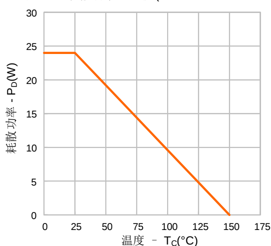
图14-1. 耗散功率vs.温度(SVS65R280FJD/FD4)
