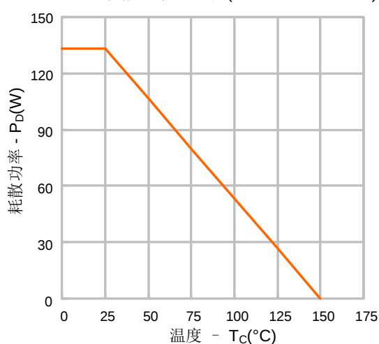
图14-3. 耗散功率vs.温度(SVS65R280T/SD4)
