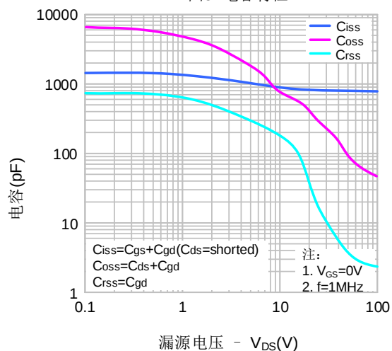
图5. 电容特性
